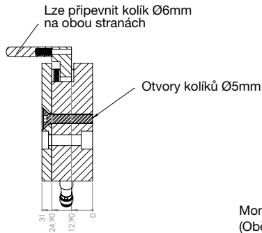
SEKCE A-A
